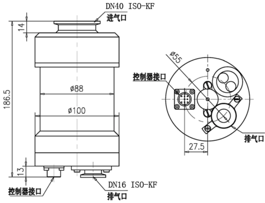
FF-40/25 外形尺寸图
