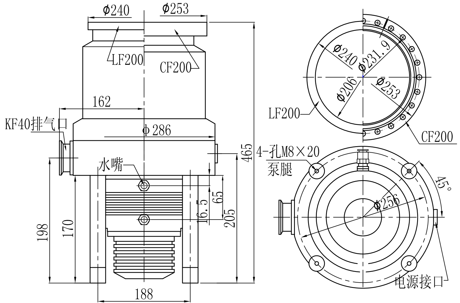
FF-200/1200C复合分子泵安装尺寸简图
